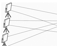
Цветные тени
